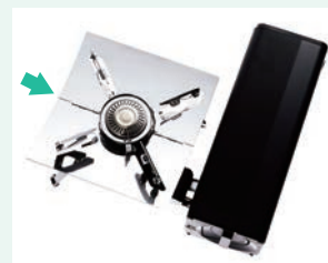
ケース背部に収納されていた、ヒートシールドを設置
