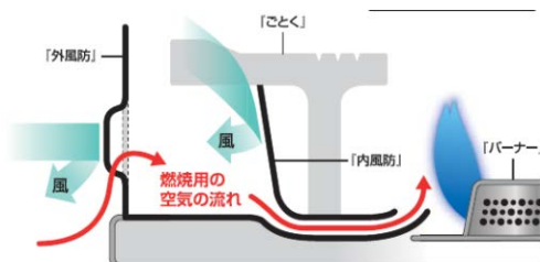
▲風は遮断しつつ燃焼用の空気は取り込む仕組み
