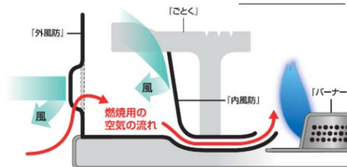
▲風は遮断しつつ燃焼用の空気は取り込む仕組み
