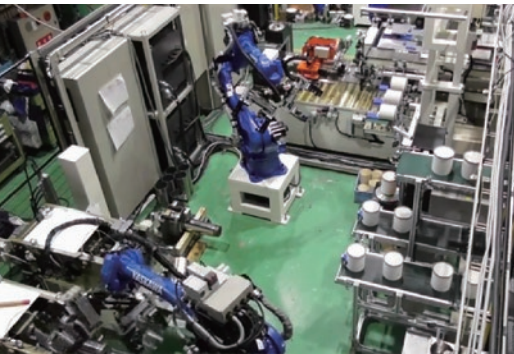
自動車排気系統部品の自動組立ロボット
